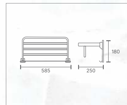
Vắt khăn giàn/ Towel rack Mã sản phẩm/ Code no.: T1209.09
