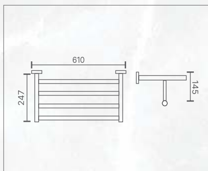
Vắt khăn giàn/ Towel rack Mã sản phẩm/ Code no.: T1309.01
