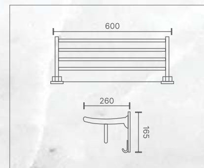
Vắt khăn giàn/ Towel rack Mã sản phẩm/ Code no.: T1309.02
