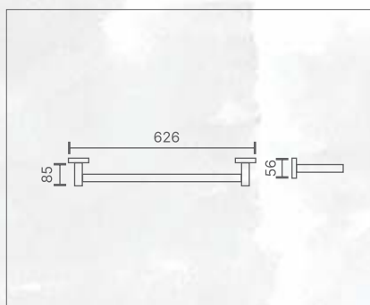
Vắt khăn đơn/ Towel bar Mã sản phẩm/ Code no.: T1307.01
